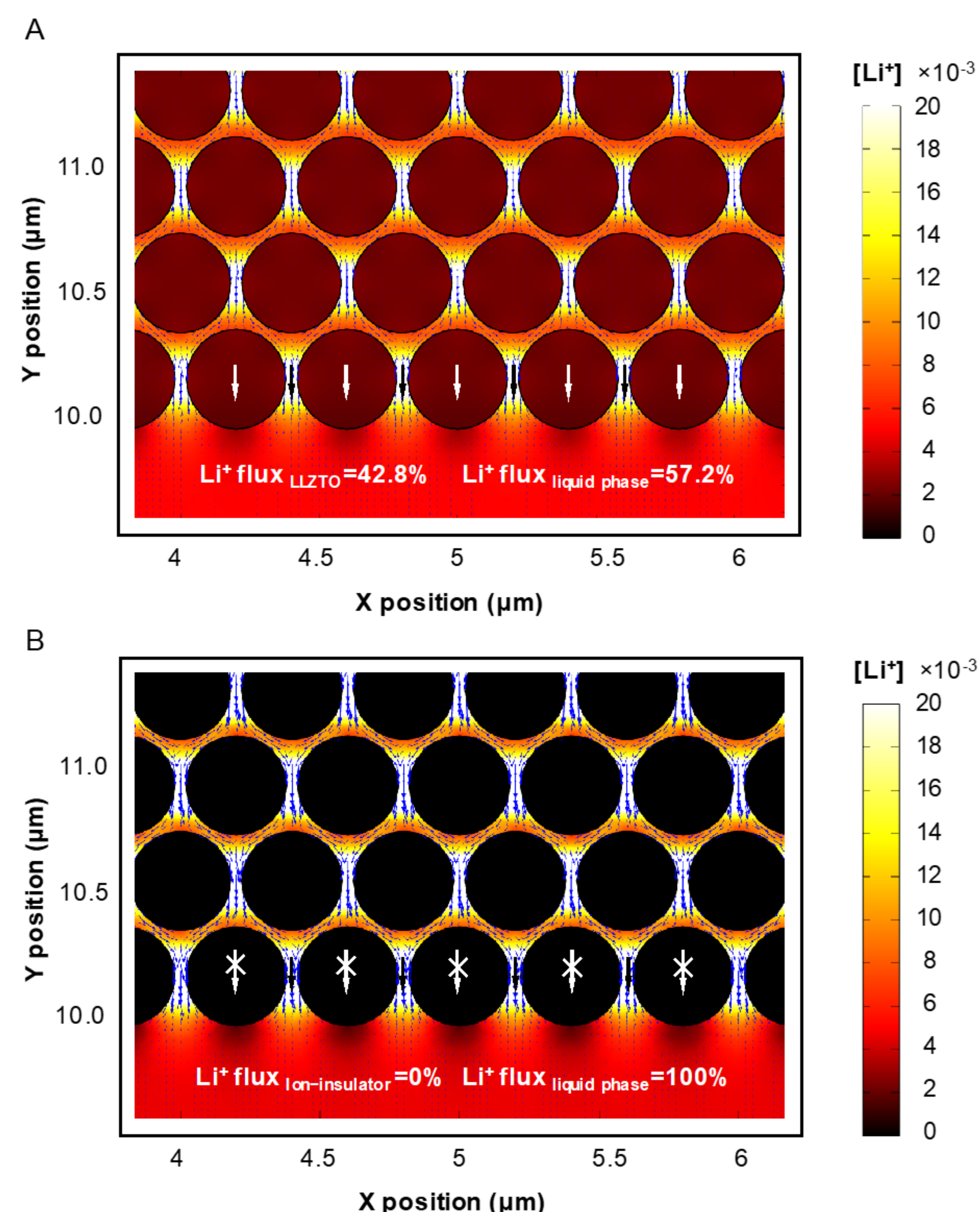
图 4. 锂离子可导的LLZTO复合隔膜与锂离子绝缘的 \text{Al}_2\text{O}_3 复合隔膜中锂离子输运通量分布
