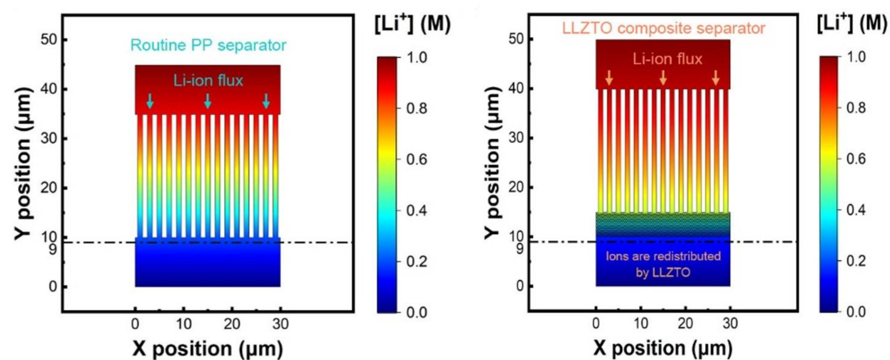
图 3. 普通PP隔膜与LLZTO复合隔膜中的锂离子浓度分布
