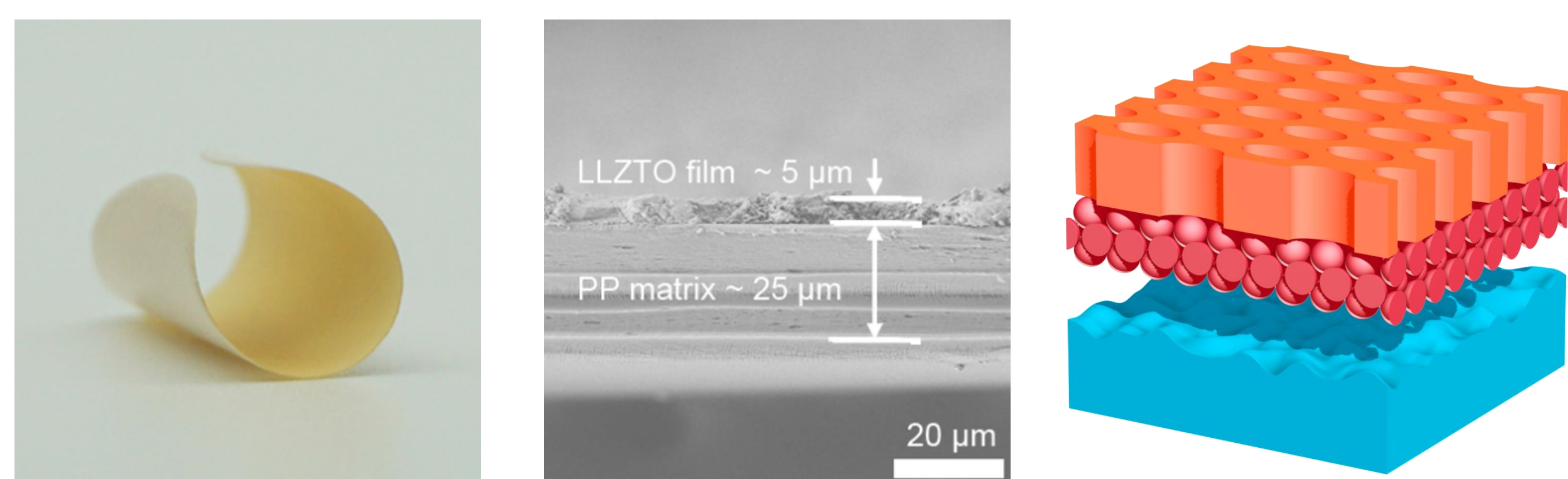
图 1. 柔性固态电解质的产品外观、SEM截面照片、结构示意图
